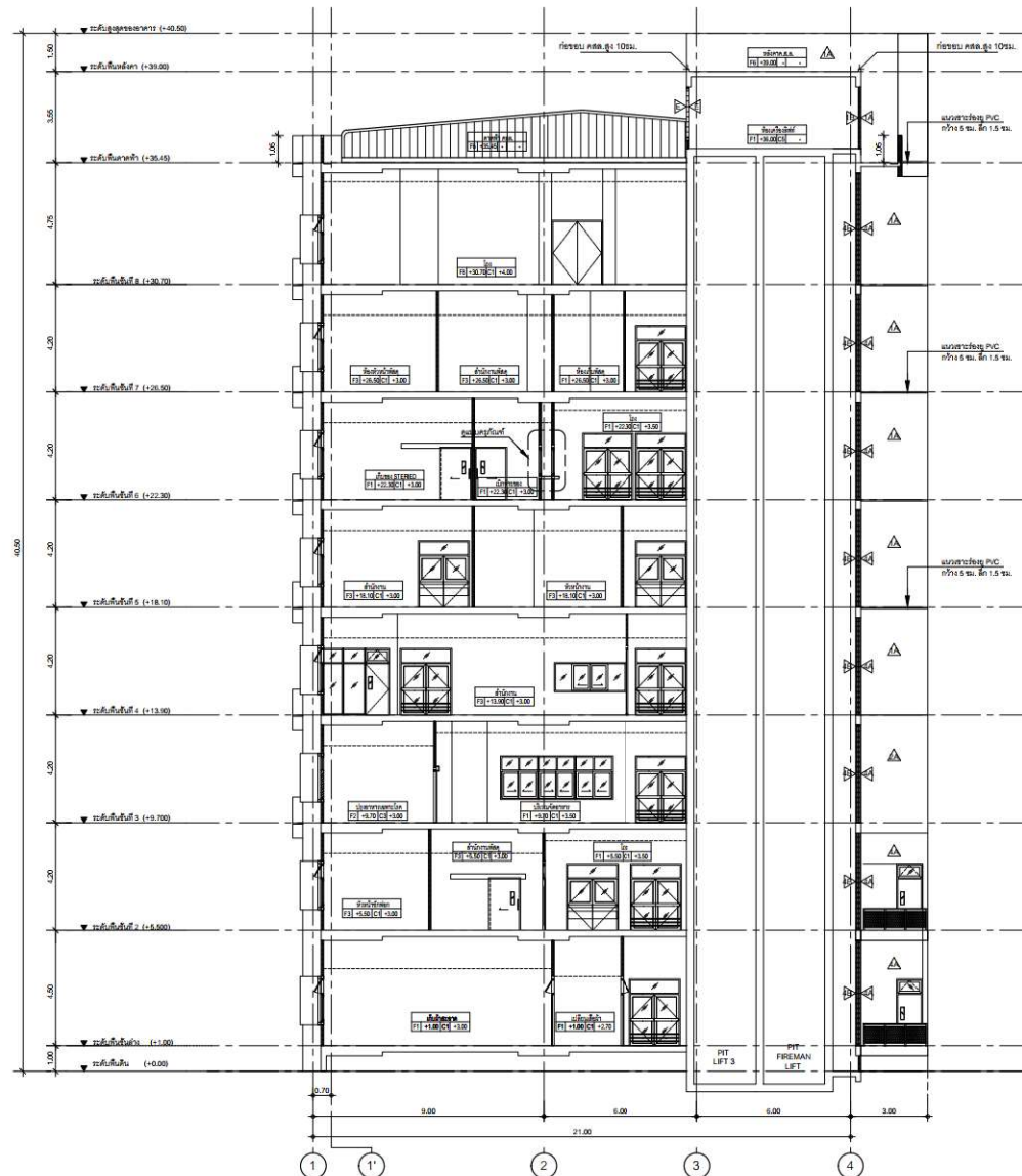
รูปตัด A มาตราส่วน 1:100
