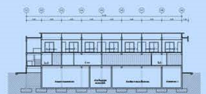
รูปตัด4
