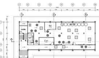
แปลนพื้นที่1
