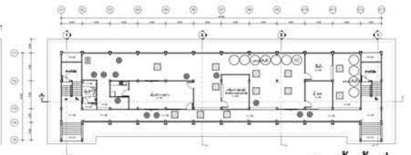
แปลนพื้นที่1
