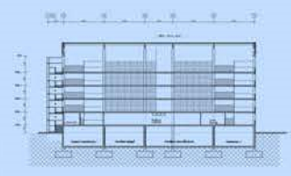
รูปตัด5
