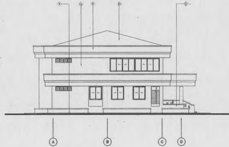
รูปด้านข้างซ้าย. มาตราส่วน 1:100
