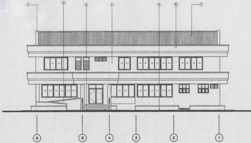
รูปด้านหน้า. มาตราส่วน 1:100
