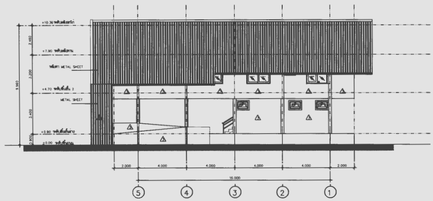
รูปตัด 3 มาตราส่วน 1:100
