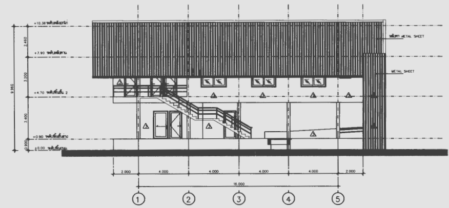
รูปตัด 1 มาตราส่วน 1:100
