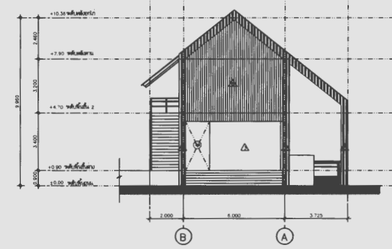
รูปตัด 4 มาตราส่วน 1:100
