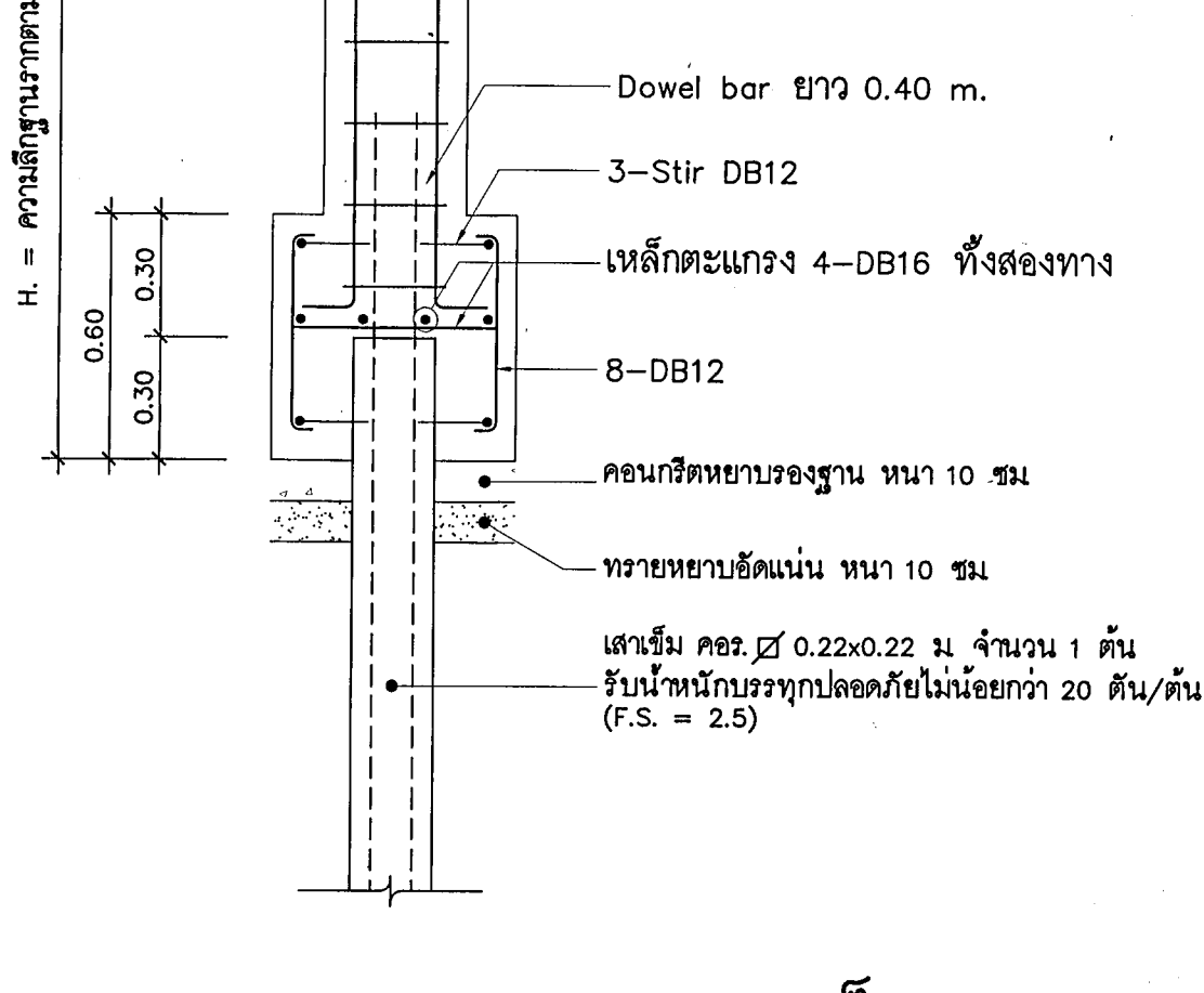
แปลนคานารับโครงหลังคา มาตราส่วน 1:20
