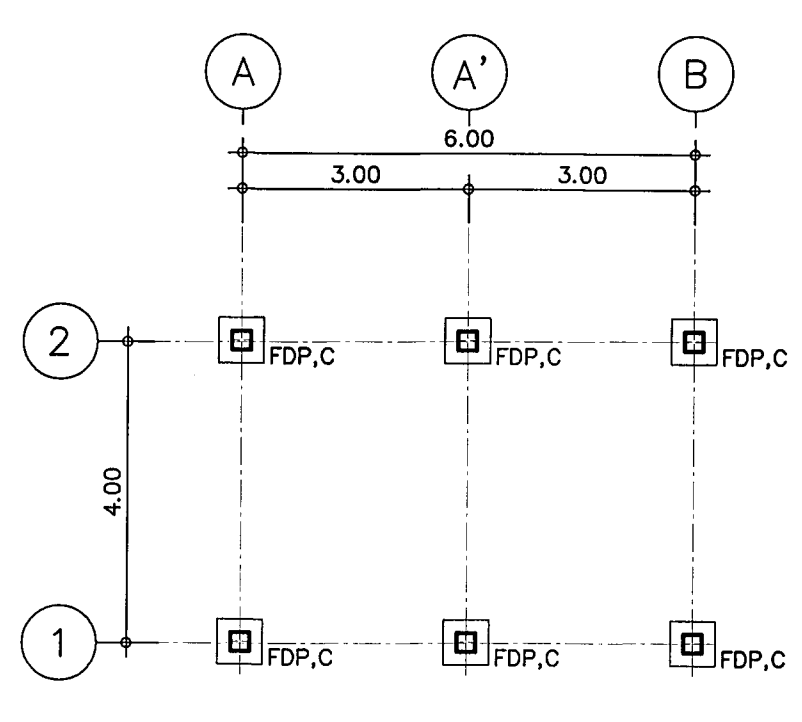
แปลนคานารับโครงหลังคา มาตราส่วน 1:100
