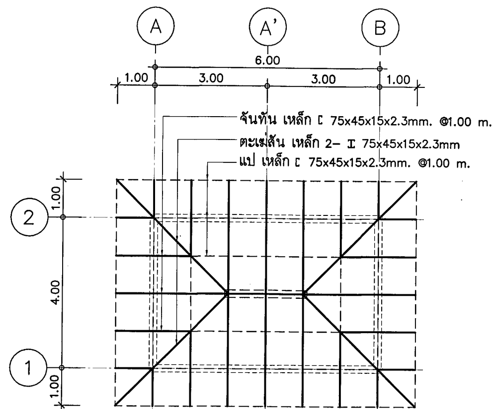
แปลนโครงหลังคา มาตราส่วน 1:100
