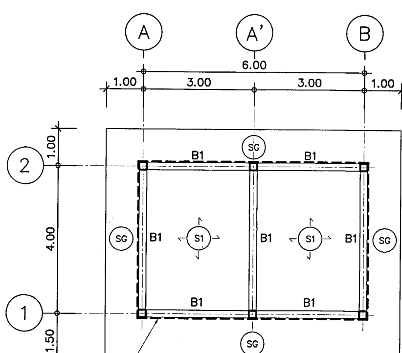
แปลนคานารับโครงหลังคา มาตราส่วน 1:100
