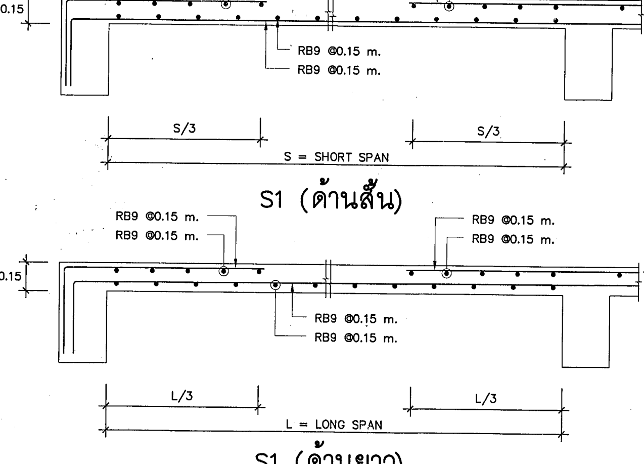
แปลนคานารับโครงหลังคา มาตราส่วน 1:20
