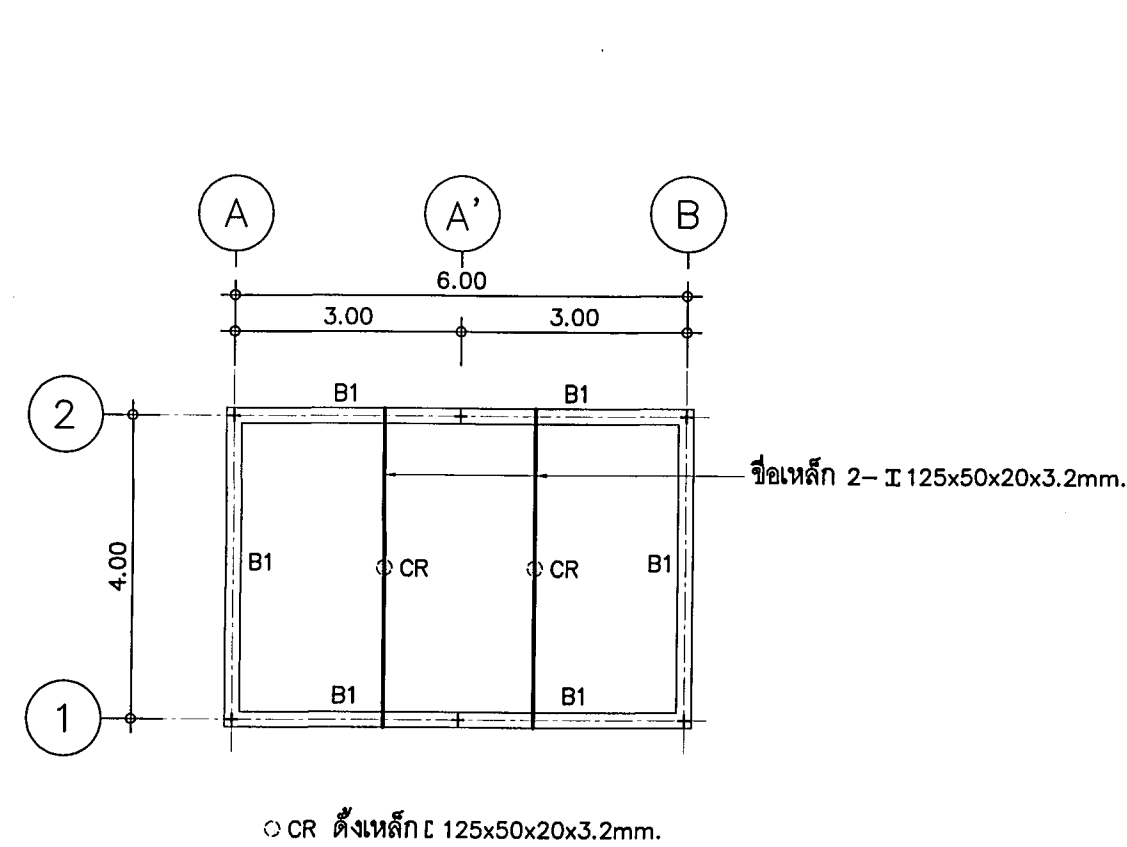
แปลนคานารับโครงหลังคา มาตราส่วน 1:100
