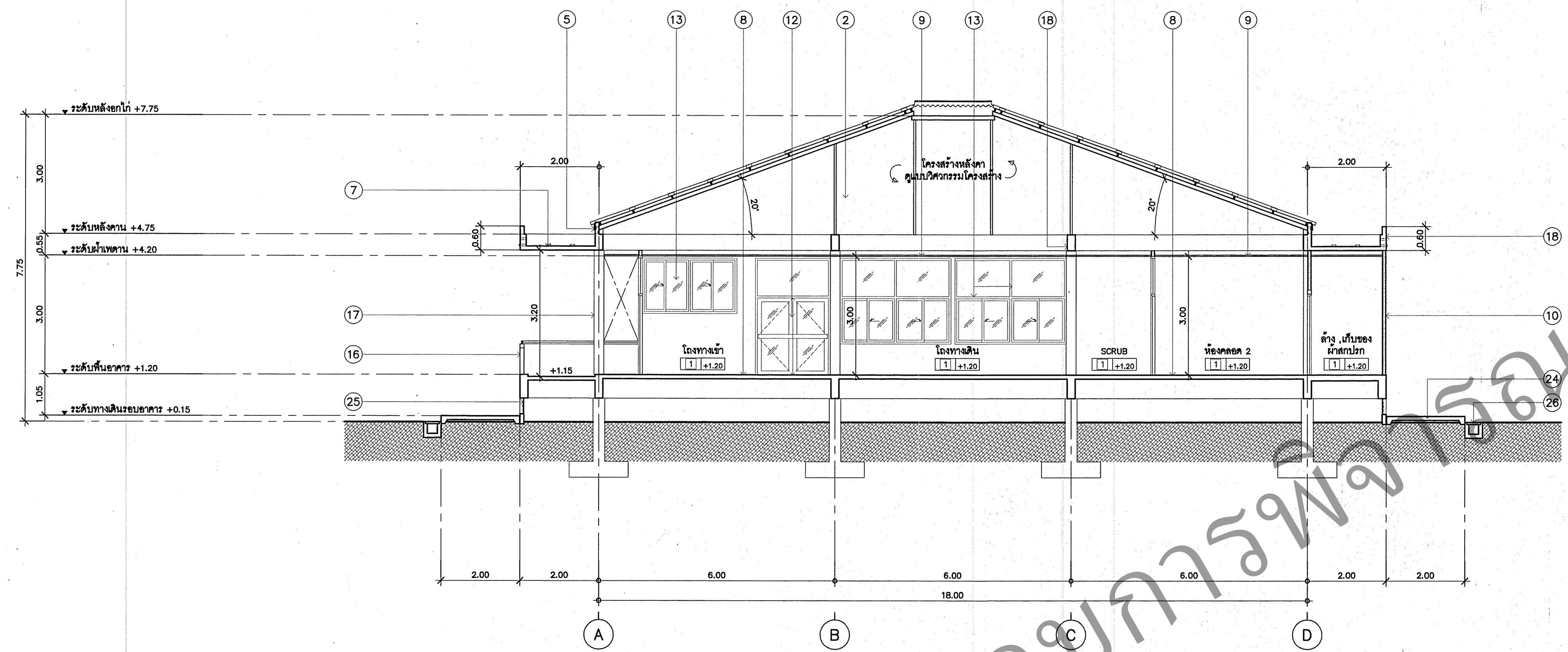
รูปตัด A-A มาตราส่วน 1:75
