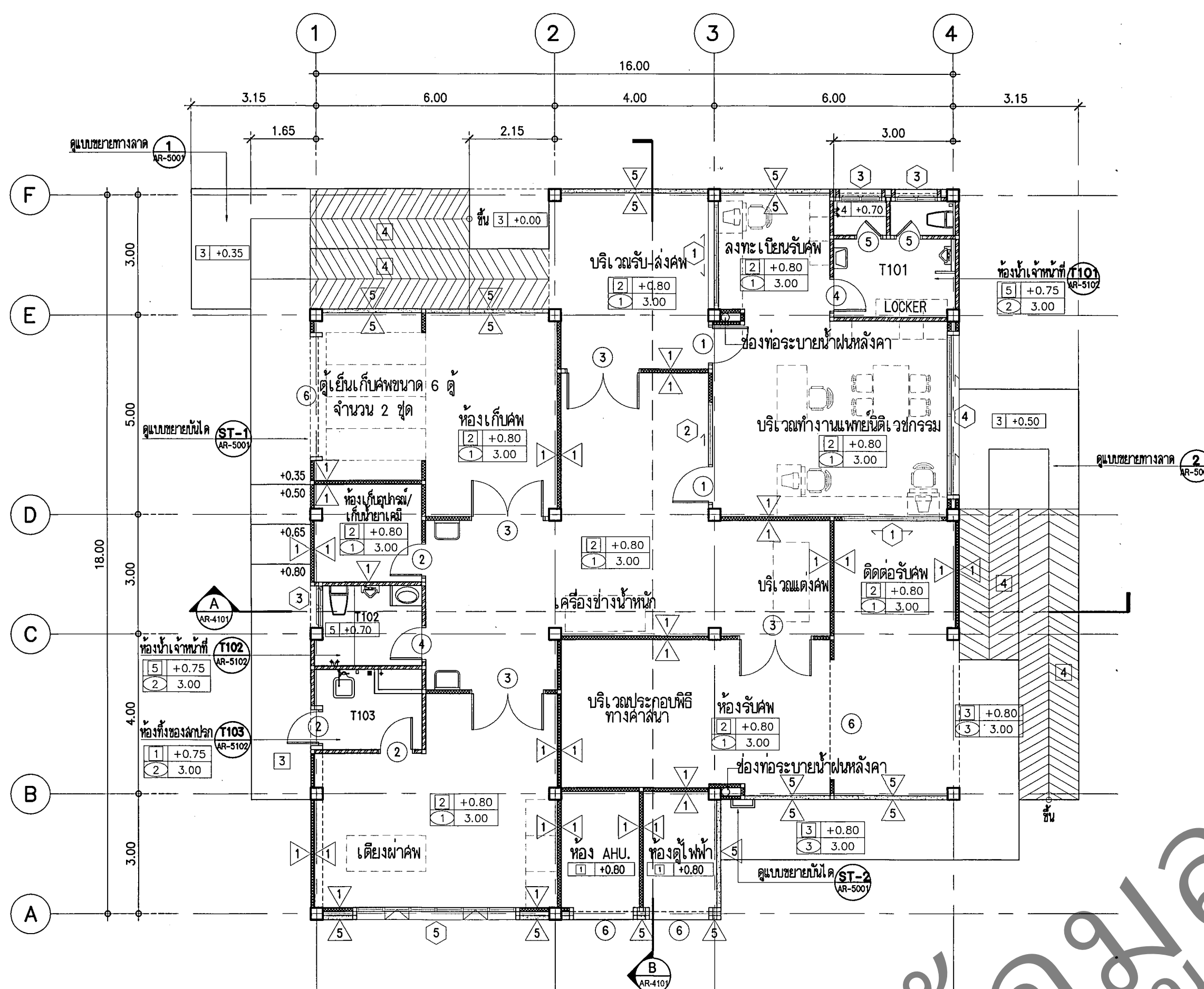
แปลนพื้นที่กลาง มาตราส่วน 1:100
