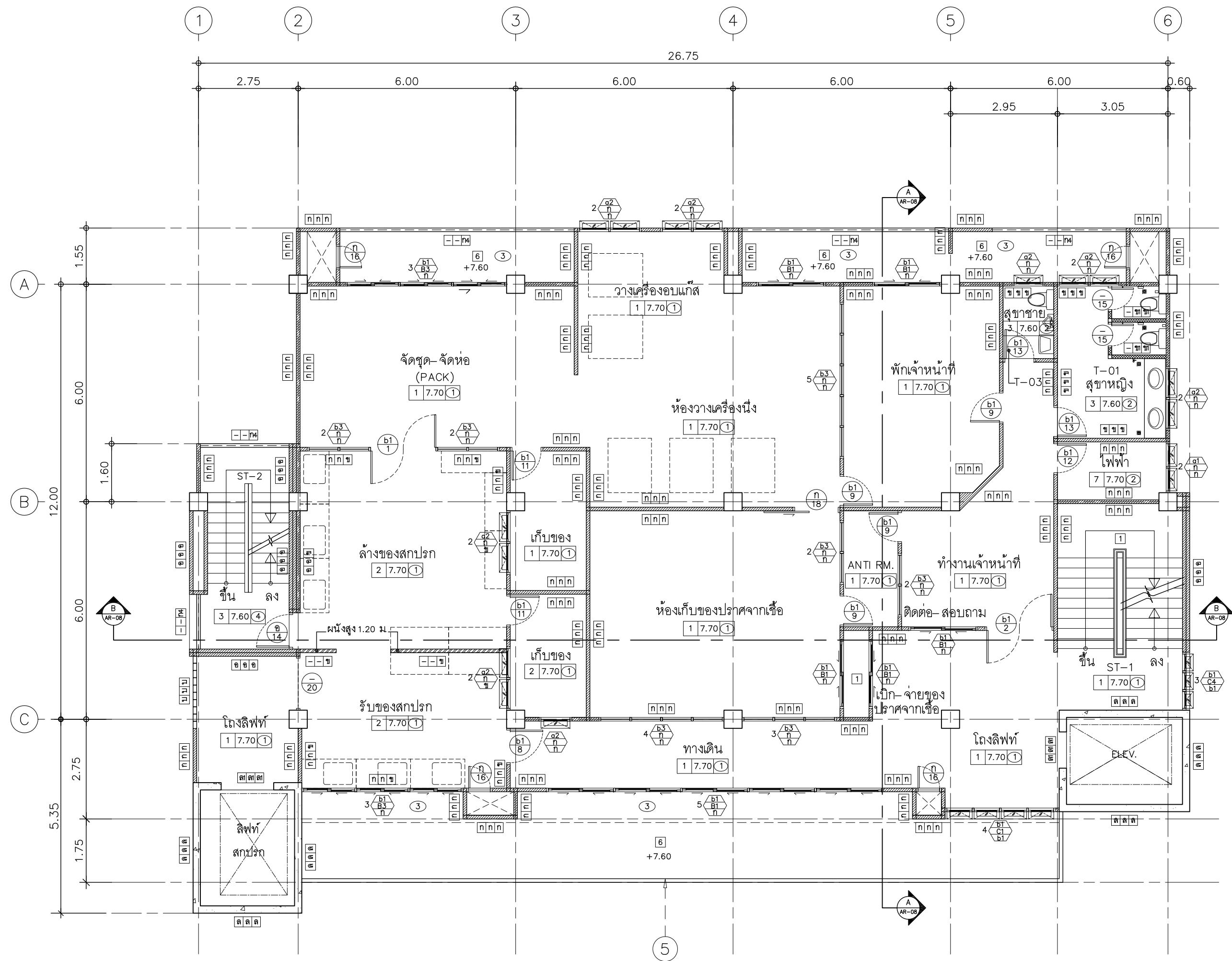
แปลนพื้นที่ 3 มาตราส่วน 1 : 100
