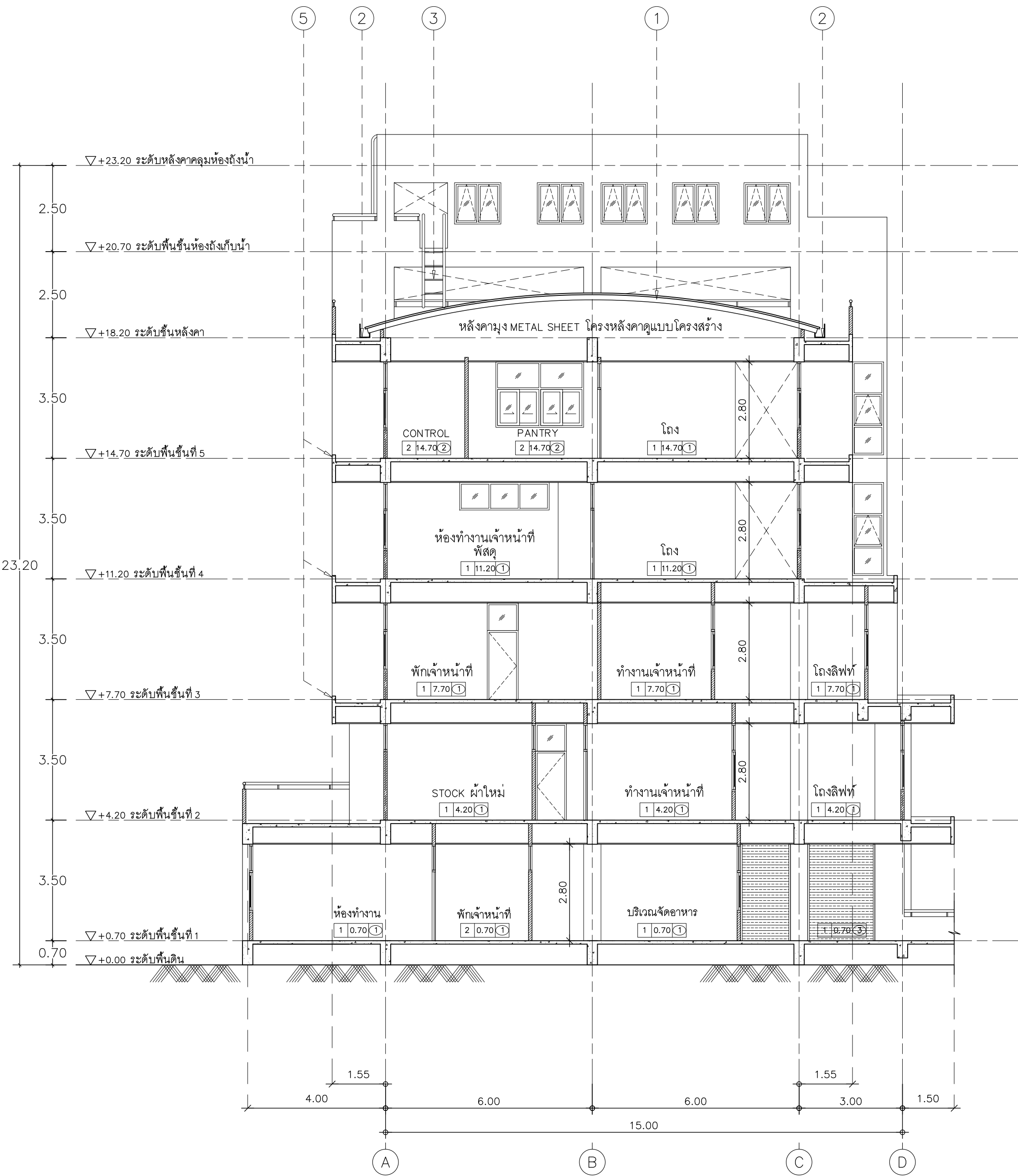
รูปตัด A-A มาตราส่วน 1: 100
